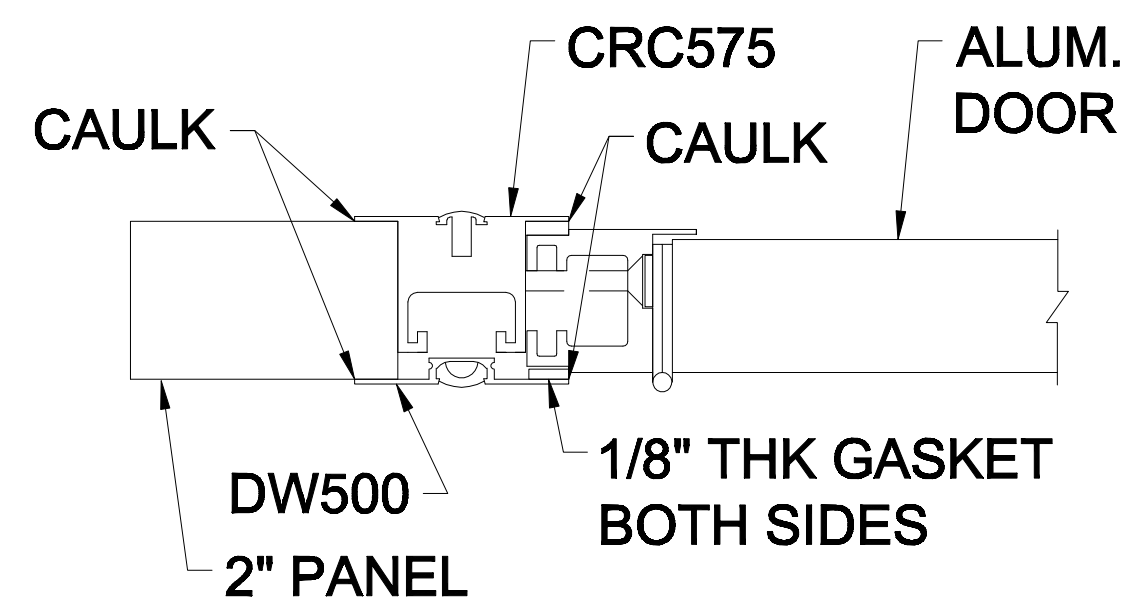
9 DOOR FRAME DETAIL N/A
